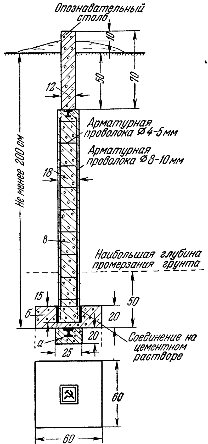
Рис. 2. Центр геодезического пункта для районов глубокого промерзания грунта (свыше 1,5 м). Тип 2
