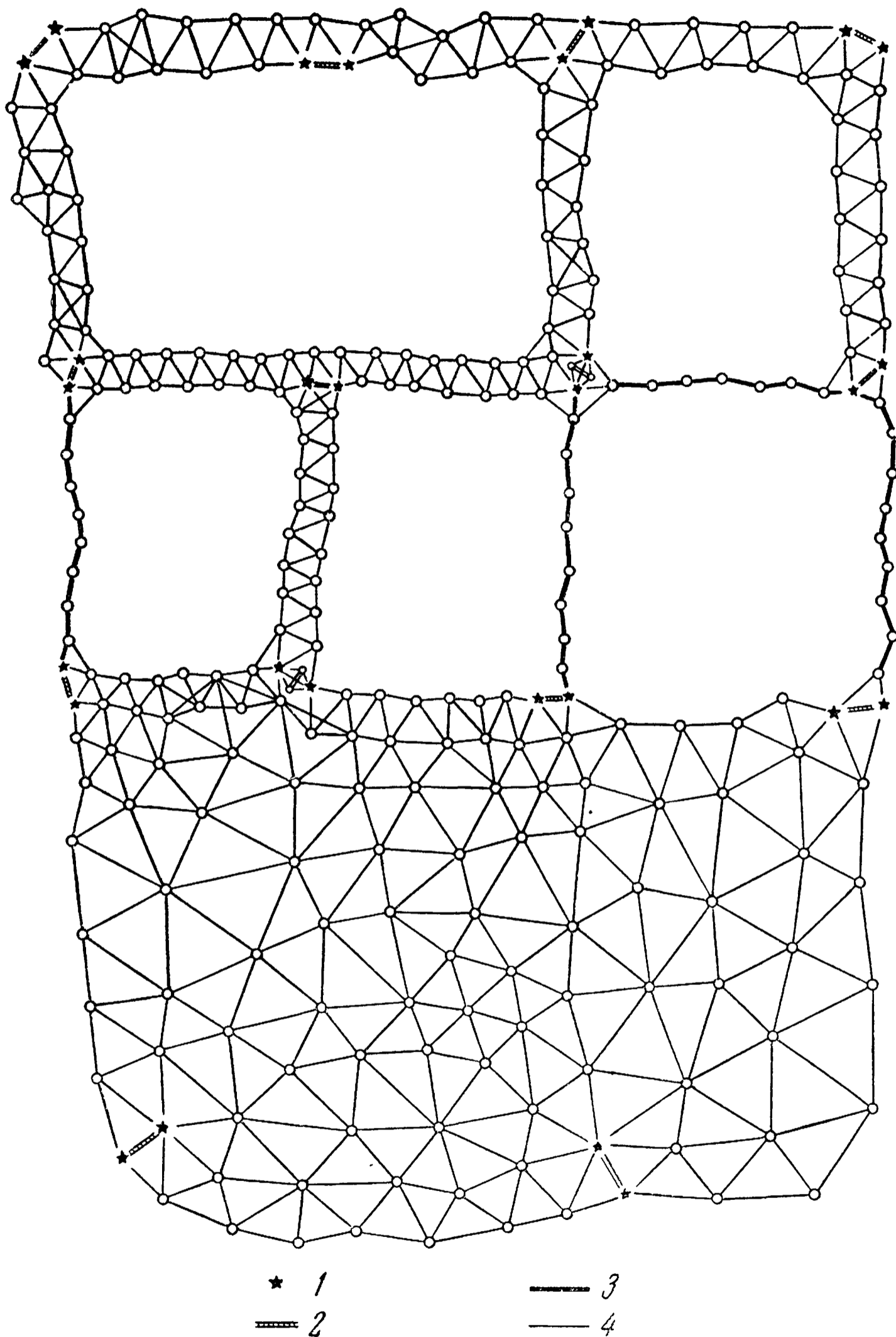
Рис. 1. Схема астрономо-геодезической сети
